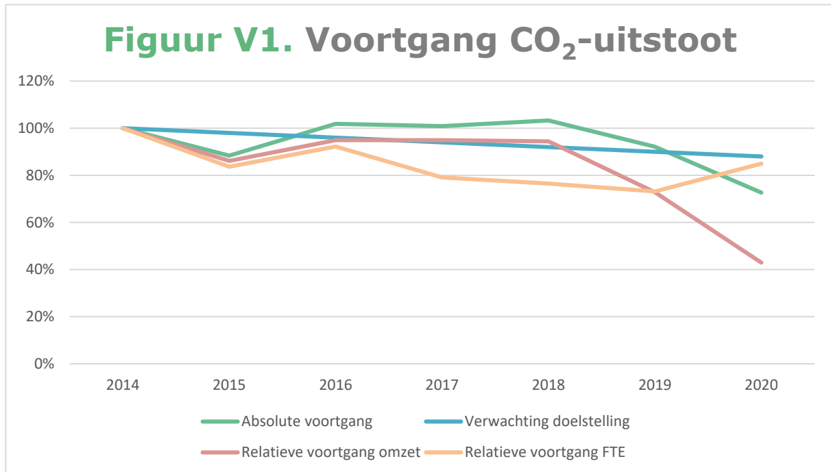
Grafiek 1: Voortgang van de CO 2 -uitstoot.
